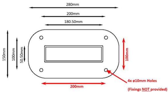
Baseplate
