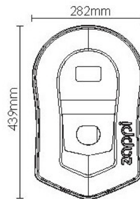
zappi dimensions
